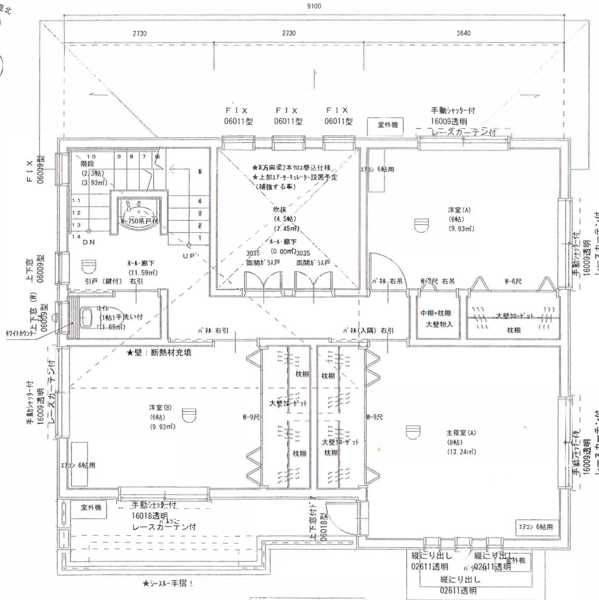
2階平面図 1/50
