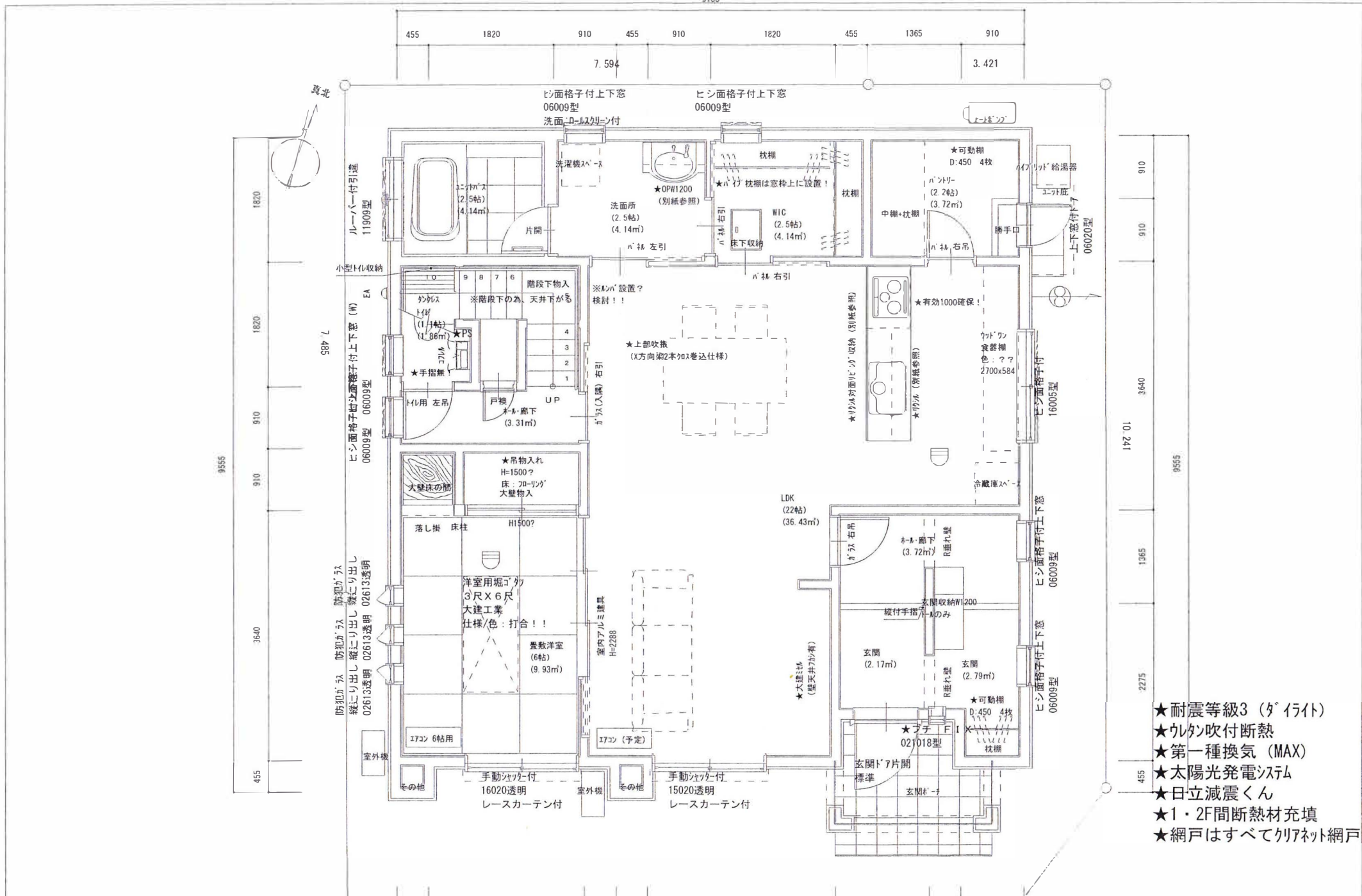
1階平面図
